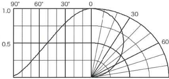
配光特性
